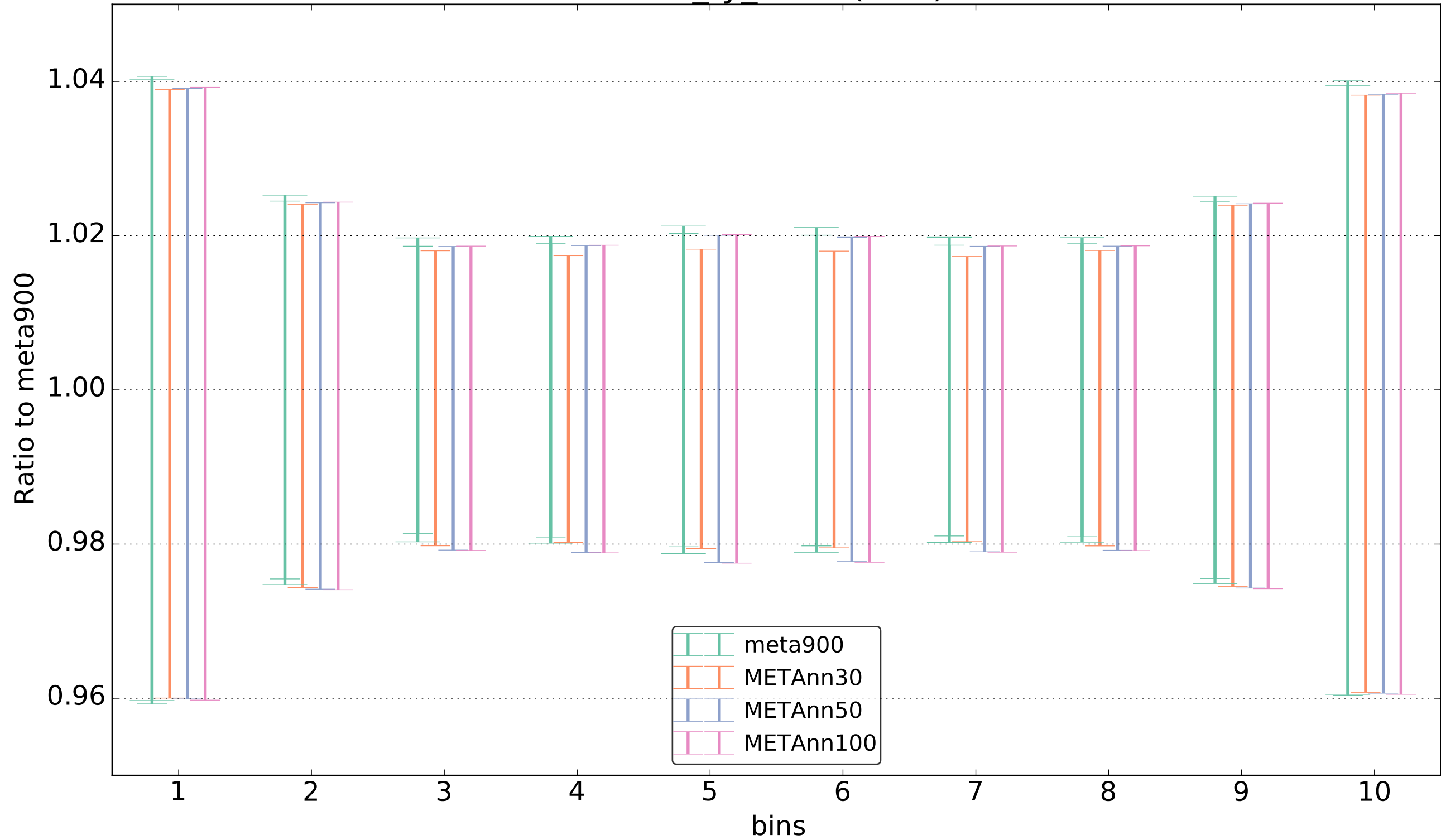
ttbar_ty_13tev(NLO)
