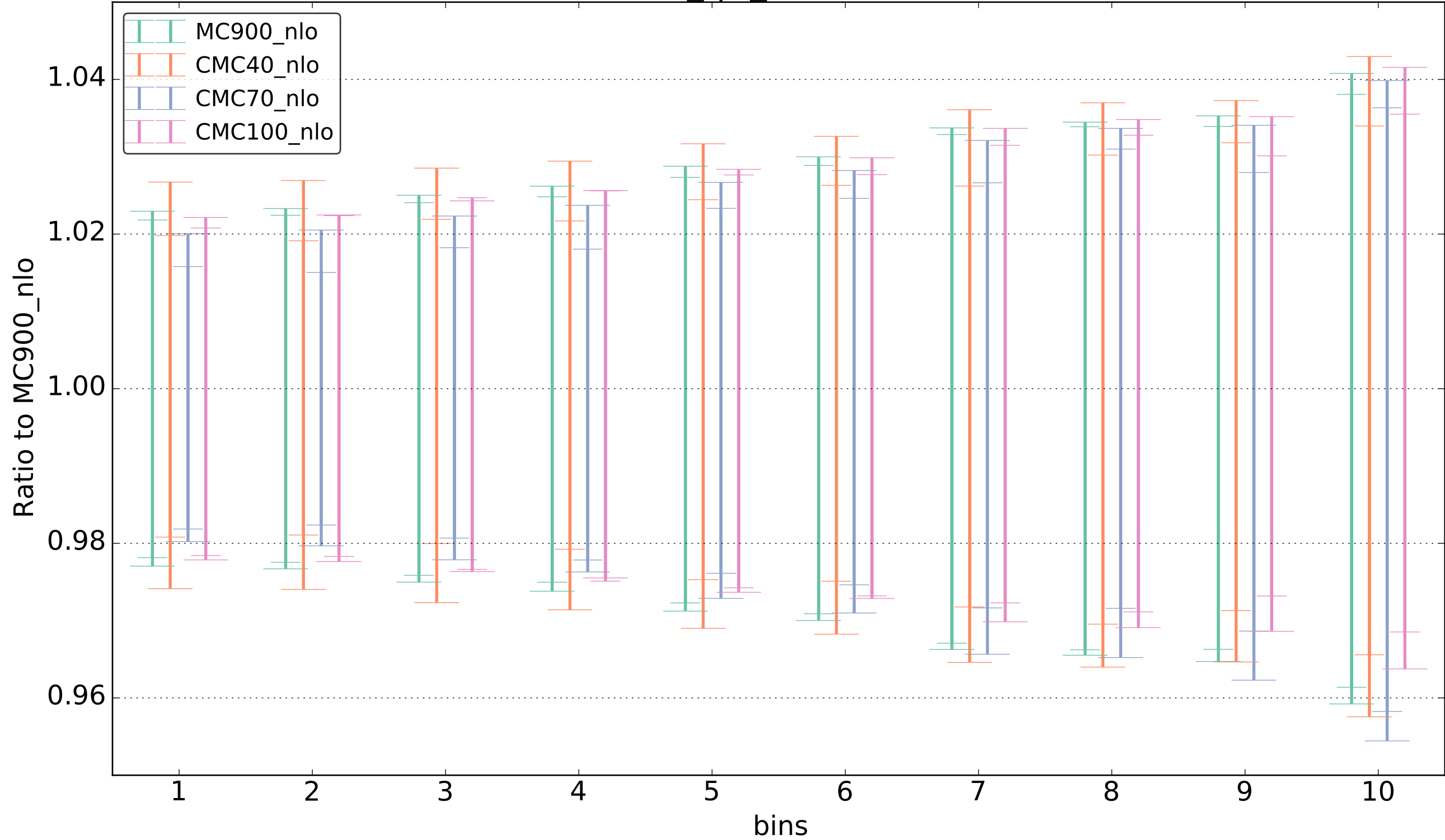
ttbar_tpt_13tev(NLO)
